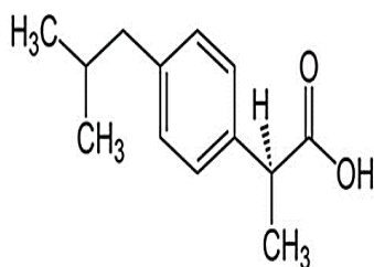
Fig. 1: Dexibuprofen
